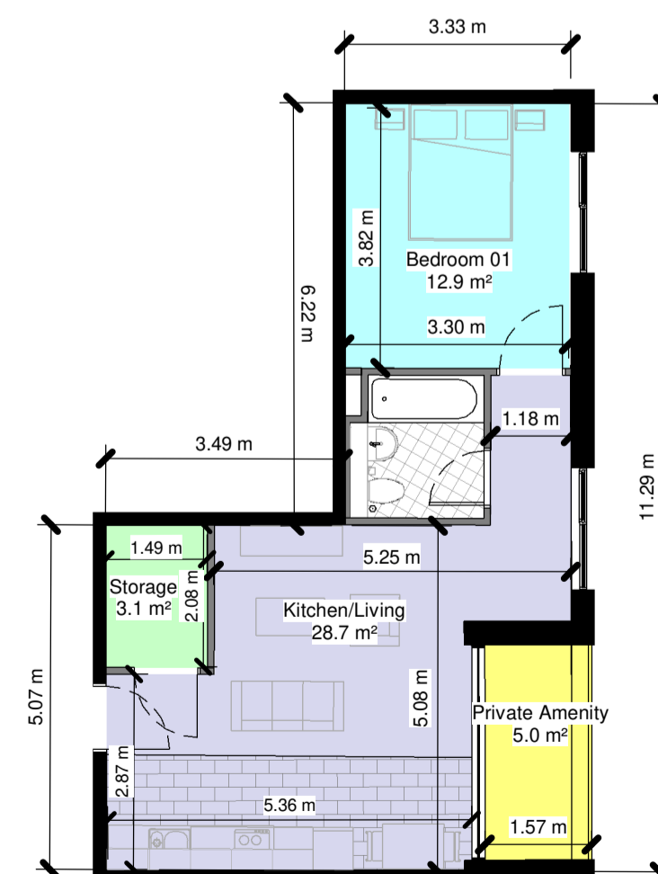
1 Bed - Type 1.22 1 : 100
