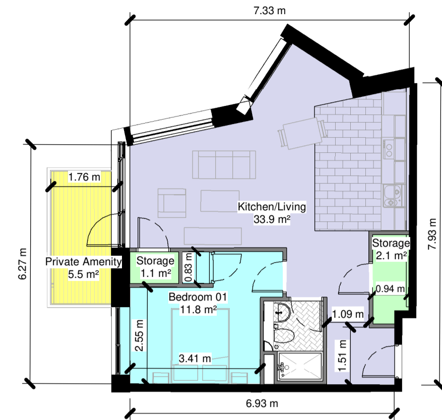
1 Bed - Type 1.13 1 : 100
