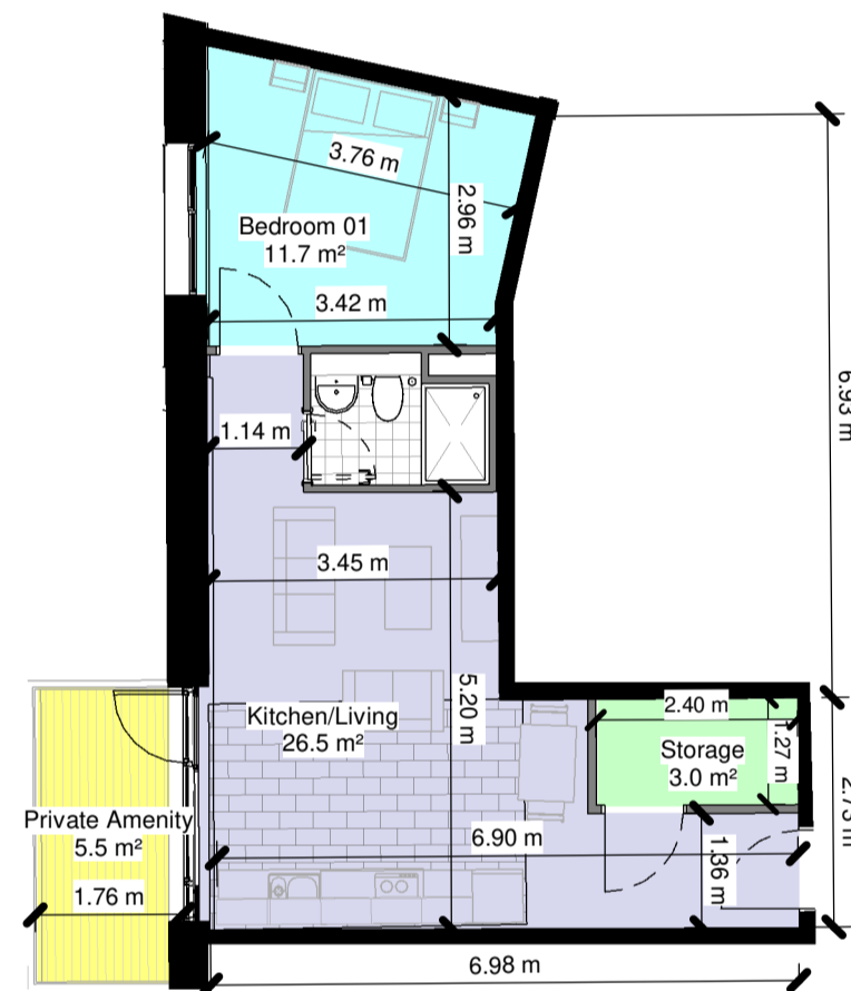
1 Bed - Type 1.17 1 : 100
