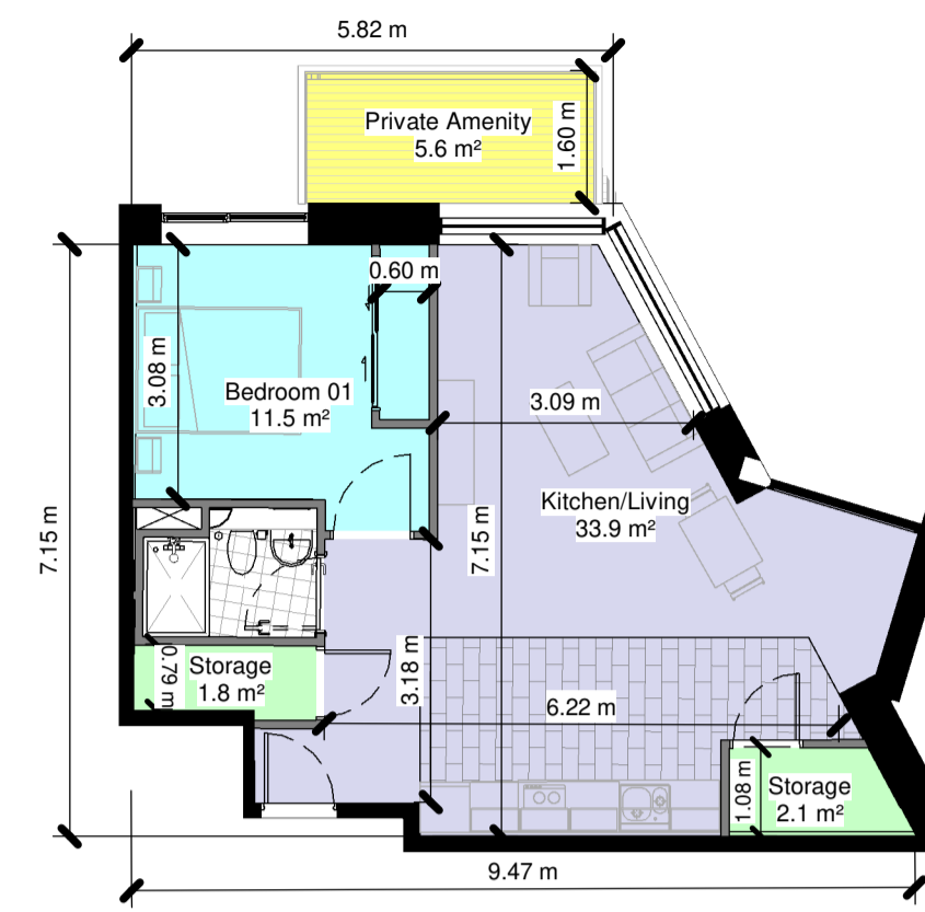
1 Bed - Type 1.15 1 : 100
