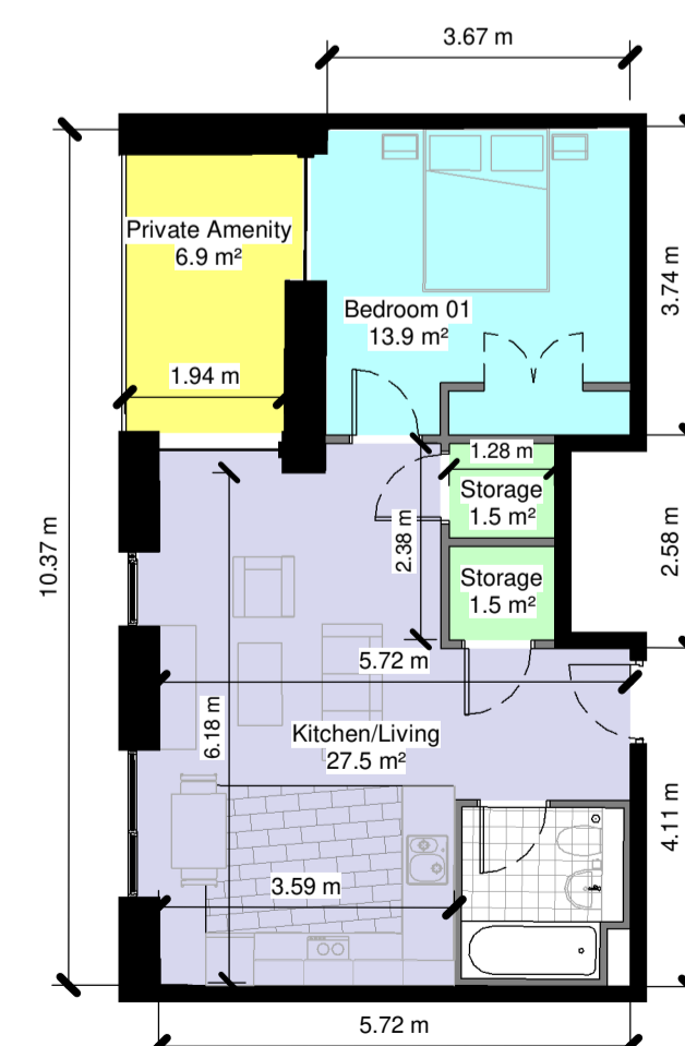
1 Bed - Type 1.23 1 : 100
