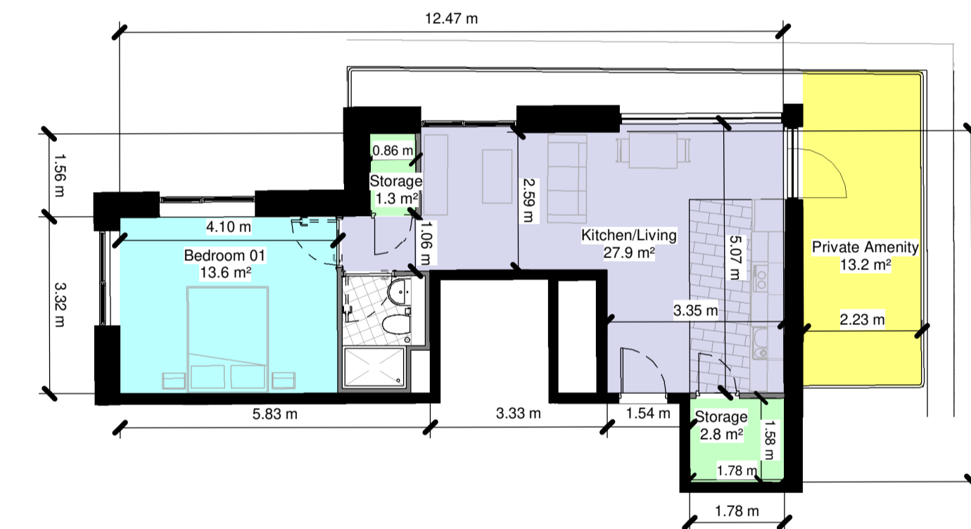
1 Bed - Type 1.20 1 : 100
