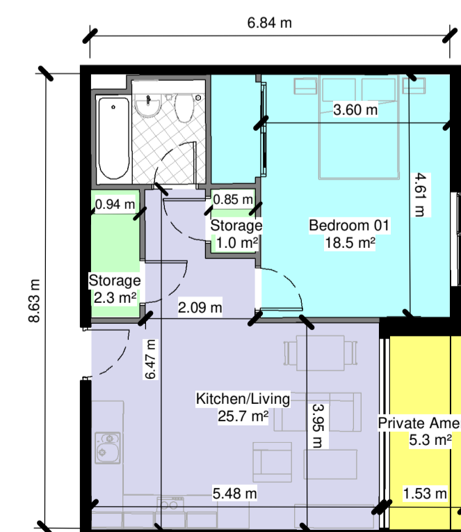
1 Bed - Type 1.24 1 : 100
