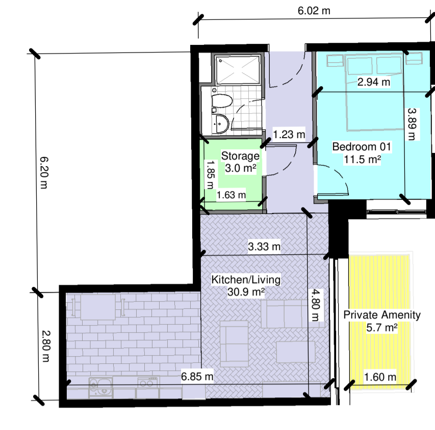
1 Bed - Type 1.16 1 : 100
