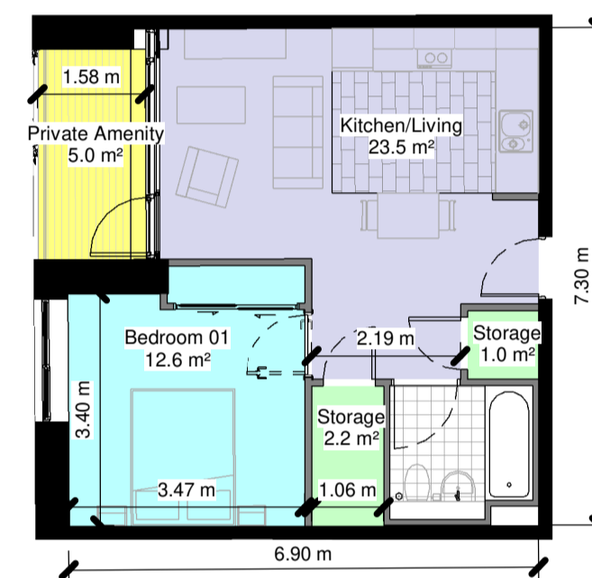
TYPE: 1.3 1 : 100
