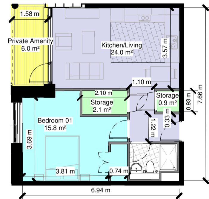
TYPE: 1.2 1 : 100
