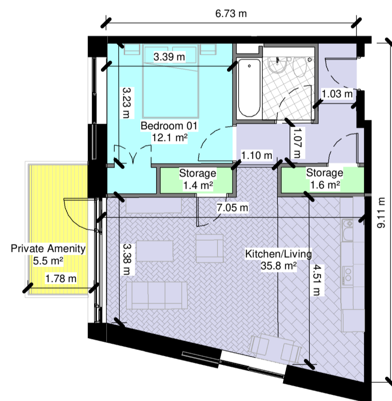
TYPE: 1.7 1 : 100
