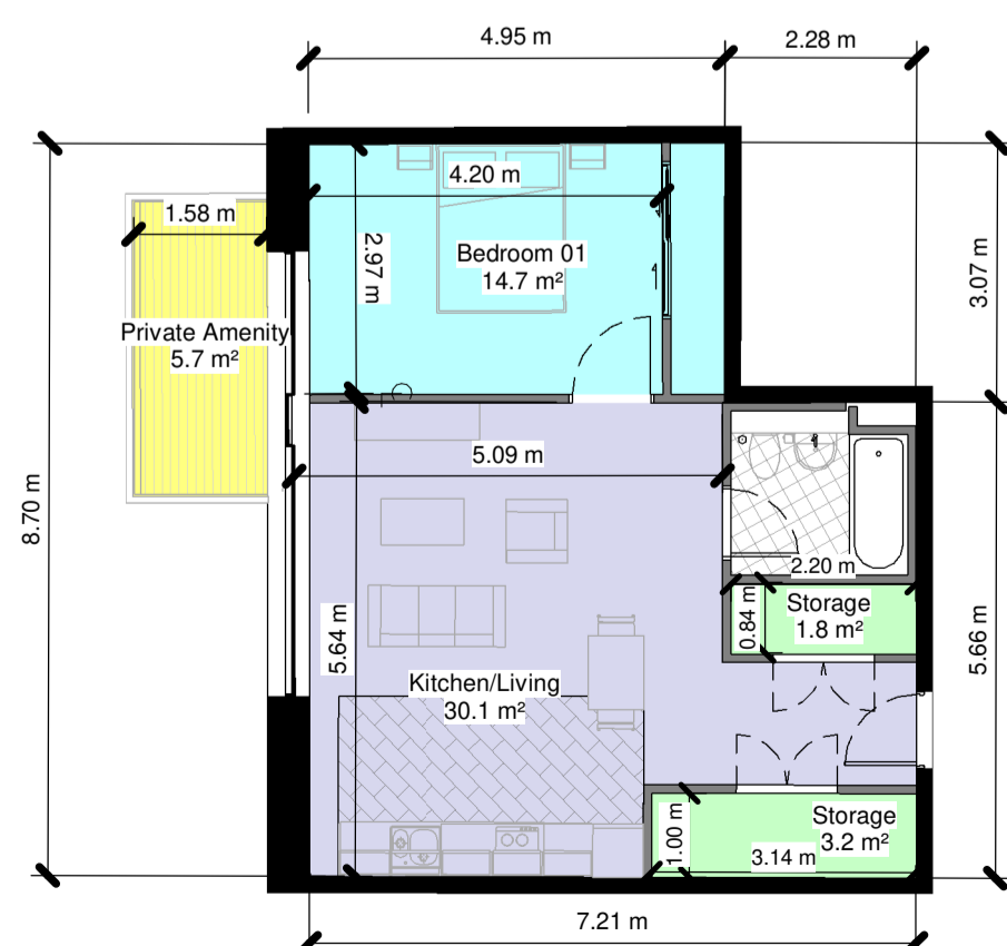
TYPE: 1.9 1 : 100
