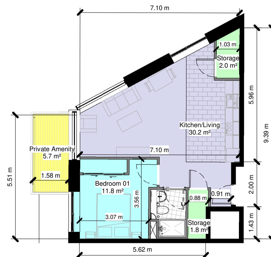
TYPE: 1.11 1 : 100
