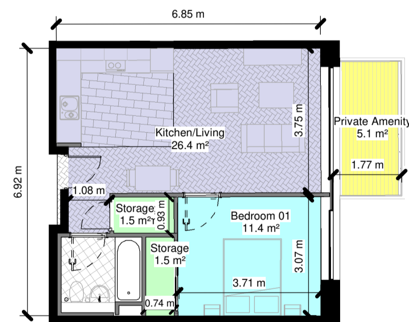
TYPE: 1.5 1 : 100
