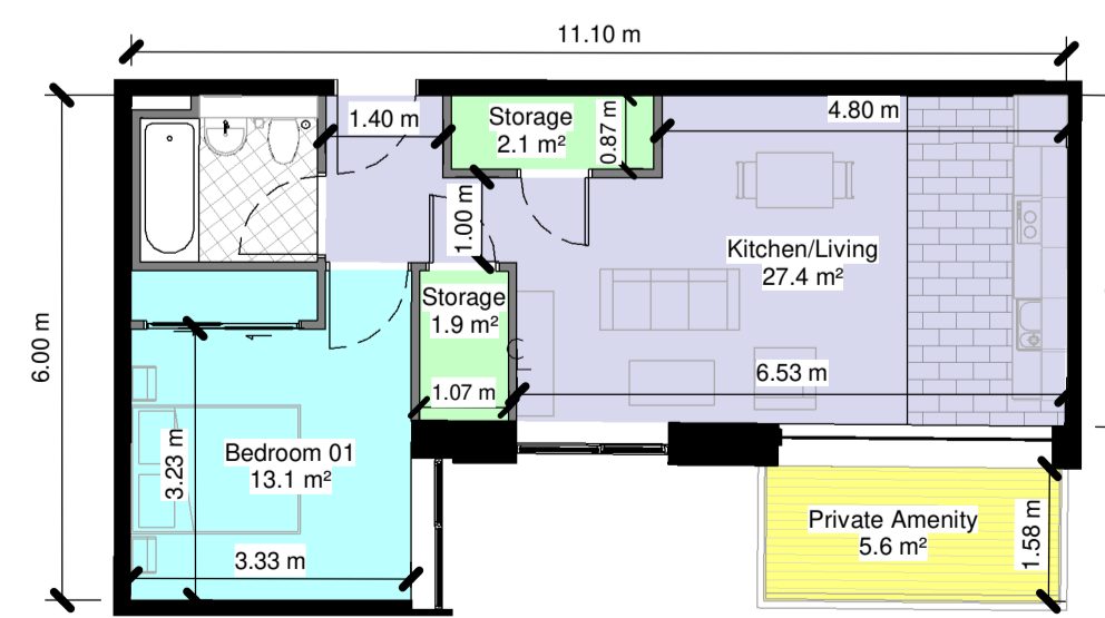
TYPE: 1.12 1 : 100
